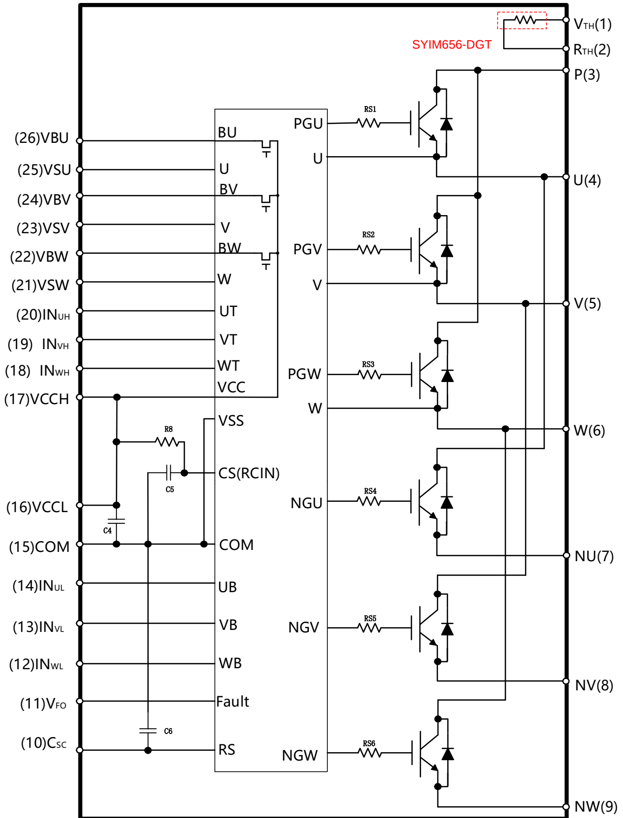
Figure1ModuleCircuitDiagram
